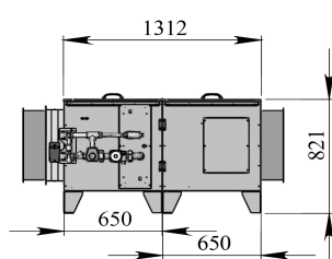
Исполнение правое, напольное Разделение на секции показано осевыми размерами
